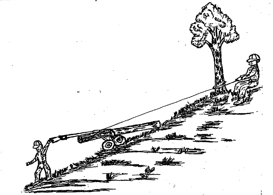
Arrastre de trozas y postes en terrenos con pendientes de hasta 45^\circ (100%)
