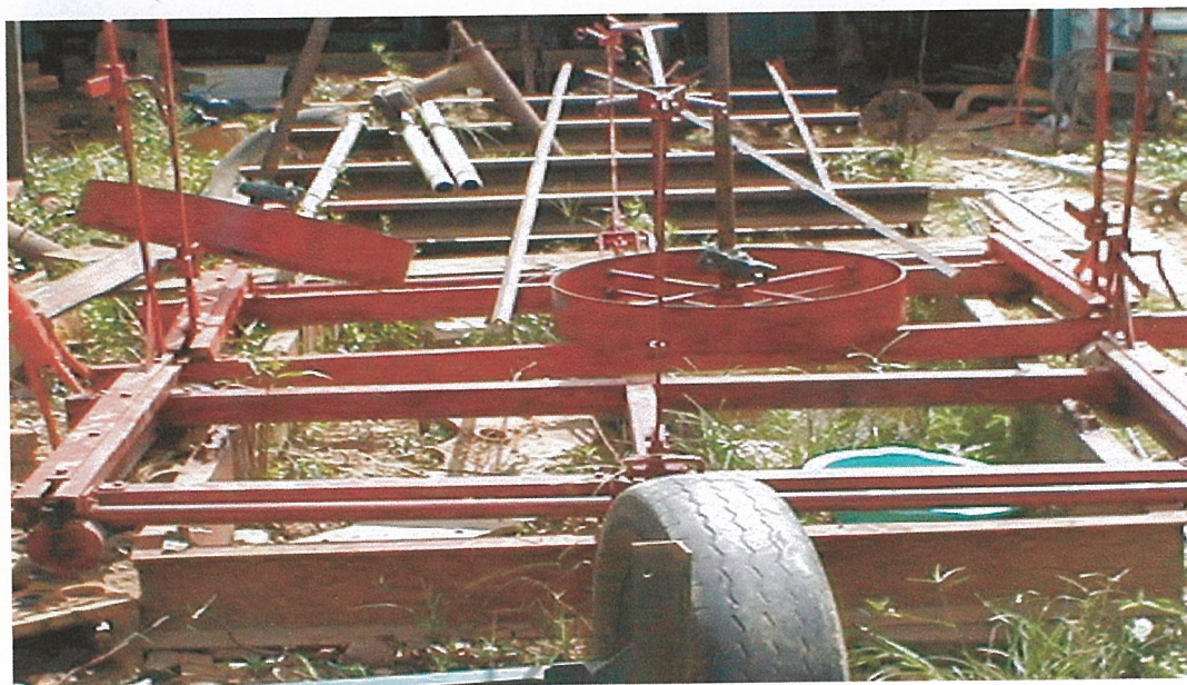
Partes y piezas de aserradero portátil de disco en taller artesanal
