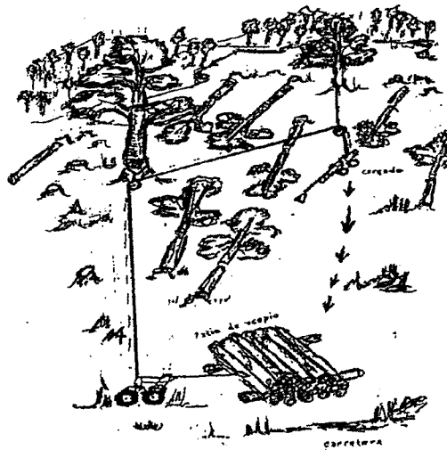
Extracción en terrenos escarpados mediante el uso de cables y poleas de cerrojo
